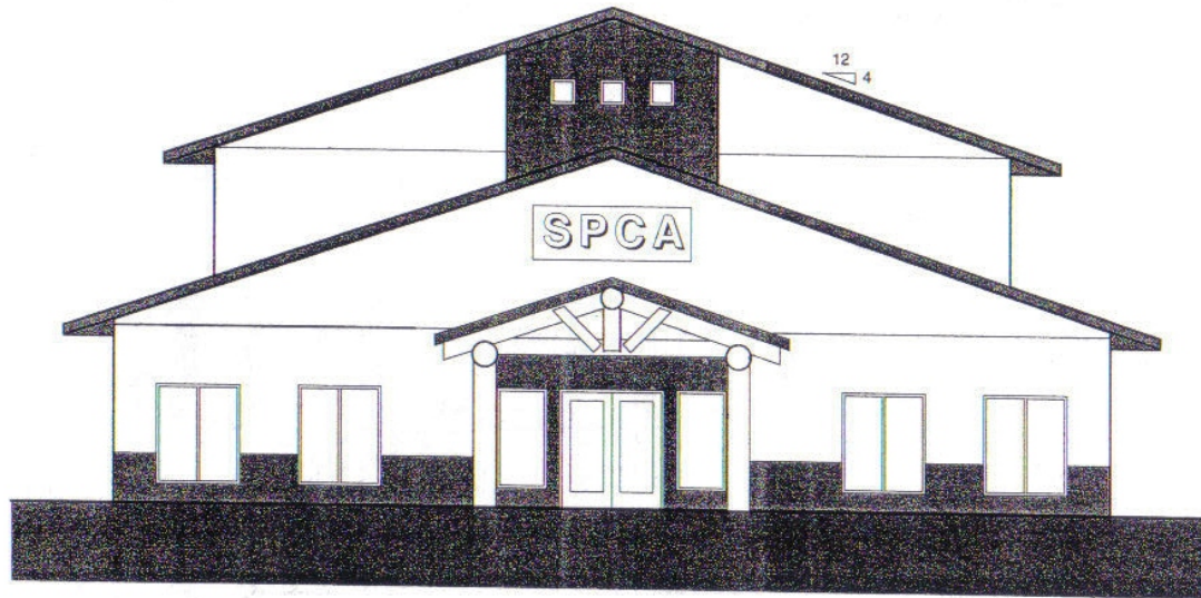
1 NORTH ELEVATION A3-01 SCALE: 1/8" = 1'-0"
